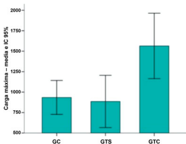
Fig. 5 Gráfico da média de carga máxima e intervalo de confiança de 95% entre os grupos estudados.
