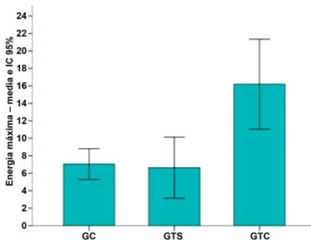
Fig. 6 Gráfico da média de energia até a fratura e intervalo de confiança de 95% entre os grupos estudados.
