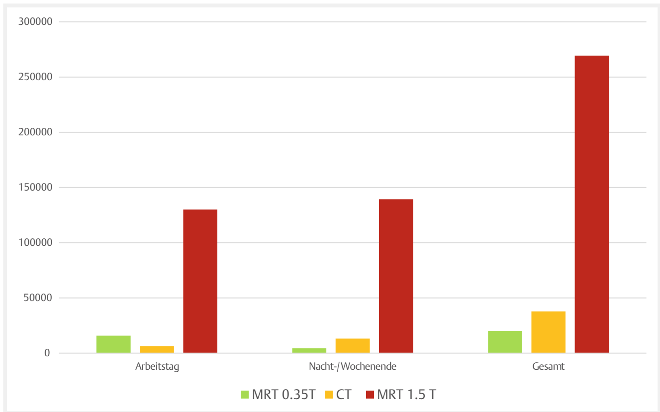
► Abb. 1 Jährlicher Energieverbrauch der Schnittbildgeräte [kWh/a]. Für Hochfeld-MRT und CT ist unter unseren Bedingungen die Leistungsaufnahme im Bereitschaftsbetrieb (Standby) aufgrund des kaum reduzierten Energieverbrauchs höher als während des Messbetriebs.
