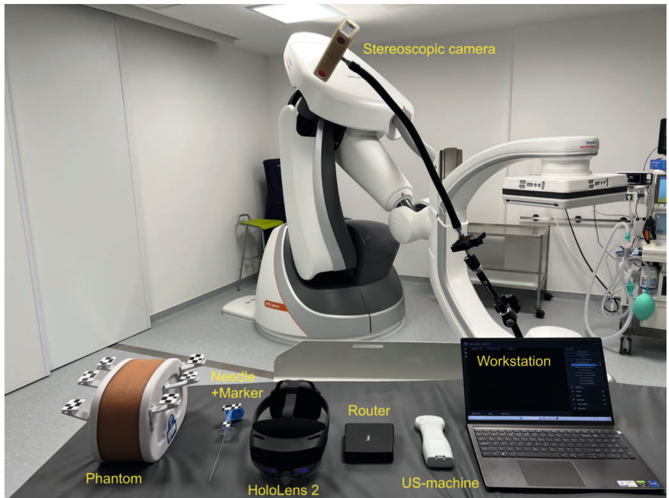
► Fig. 1 Equipment.
