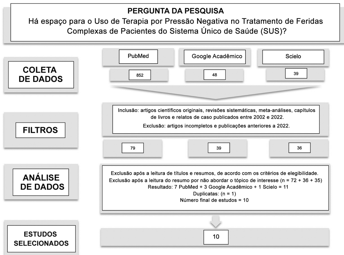
Fig. 1 Diagrama de seleção dos estudos.
